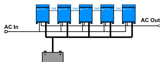
Vijf parallelle eenheden: uitgangsvermogen 12,5 kW
