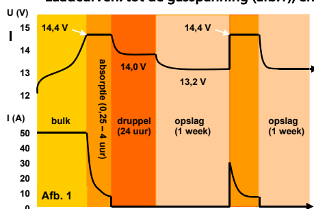
Laadcurven: tot de gasspanning (afb.1), en overschijding van de gasspanning (fig. 2)
