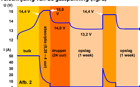
Laadcurven: tot de gasspanning (afb.1), en overschijding van de gasspanning (fig. 2)
