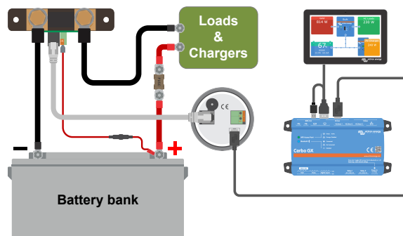
De accumonitor is verbonden met een Cerbo GX en een GX Touch scherm.
