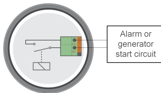
Het interne bedradingschema van de accumonitor met de relais in een buiten werking gestelde status, verbonden met een extern alarm of aggregaat startcircuit.
