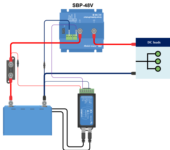
Smart BatteryProtect gebruikt de Load Disconnect van een smallBMS
