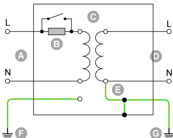
Intern bedradingsschema van de scheidingstransformator.
