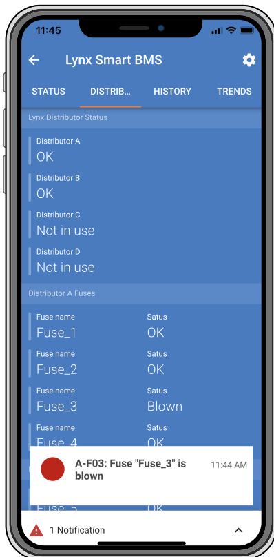
Voorbeeld van een zekeringalarm in de VictronConnect-app en een GX-apparaat
