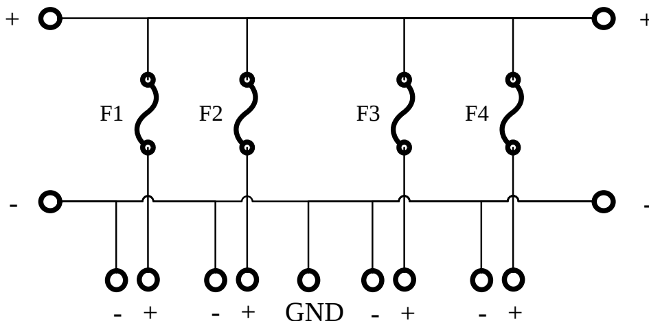
Het intern bedradingsschema van de Lynx Distributor
