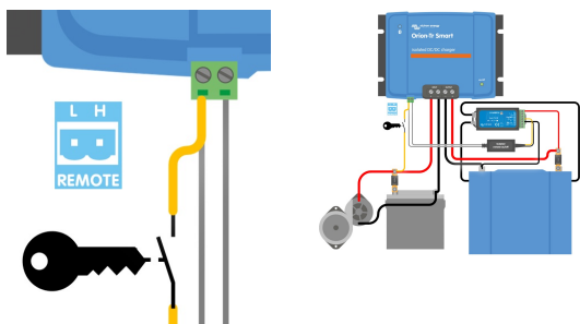
Afbeelding 4: Overschrijven detectie motoruitschakeling aansluitingsdiagram
