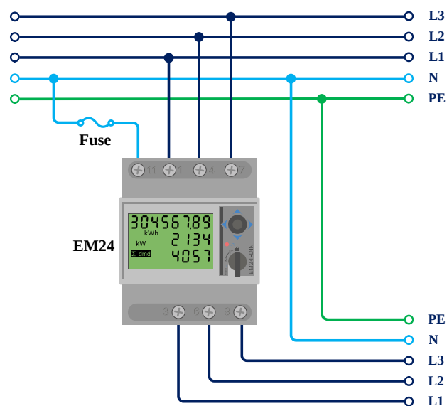
EM24-bedrading 3-fasen
