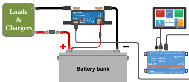
De accumonitor is verbonden met een Cerbo GX en een GX Touch scherm.
