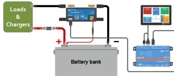
Voorbeeld van een accumonitor aangesloten op een GX-apparaat.
