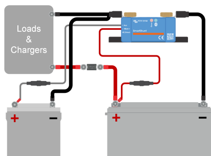
Accumonitor met bewaking reserve tweede accu.
