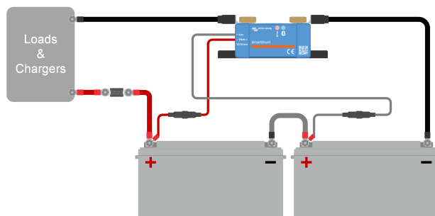
Accumonitor met reserve middelpuntbewaking.
