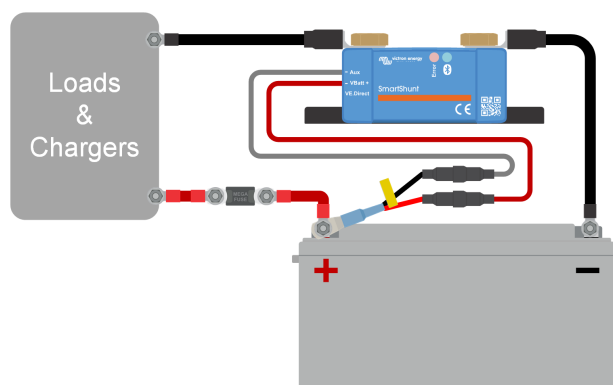
Accumonitor met reserve temperatuurdetectie.
