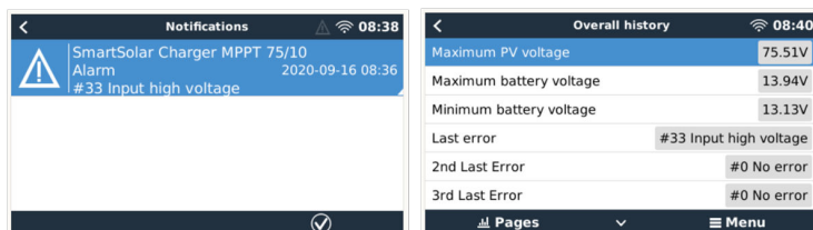
GX-apparaat met alarmmelding en historische fouten.
